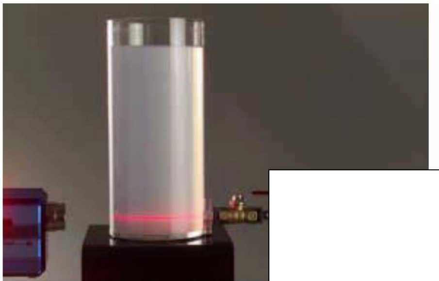
Experiência de John Tyndal (1820-1893)
